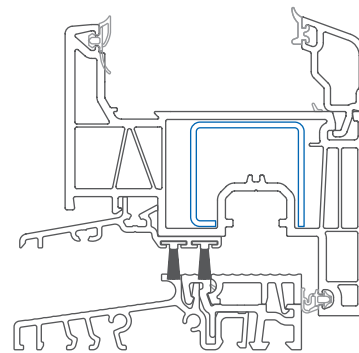
Elegant balkonska vrata s pragom sa zaobljenom letvicom ostakljenja Mjerilo: 1:2
