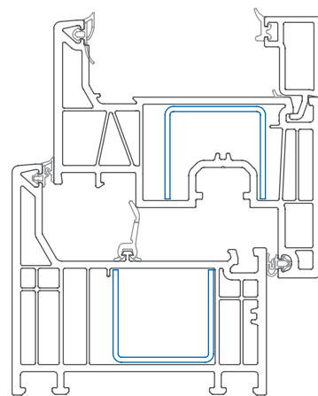
Elegant ravno krilo Okvir i krilo u zamaknutim ravninama Mjerilo: 1:2
