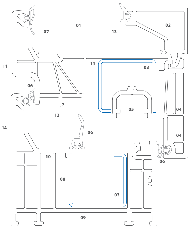
Elegant premium krilo Okvir i krilo u istoj ravnini Mjerilo: 1:1
